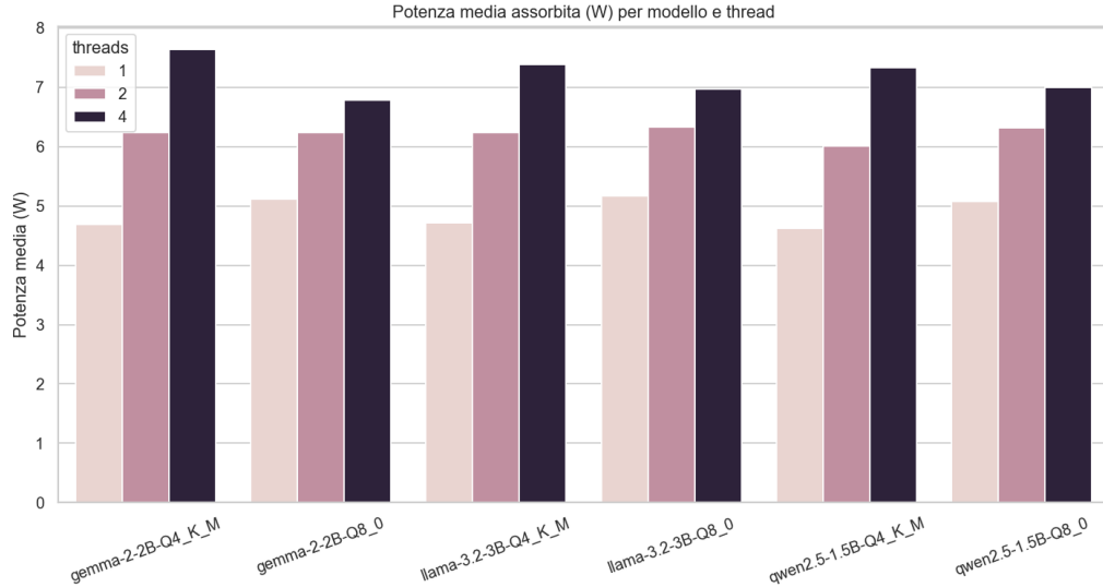
Figura 4.9: Potenza media assorbita al variare del numero di thread (Campagna B).
