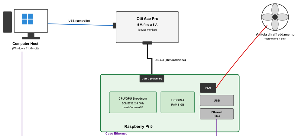
Figura 2.1: Architettura hardware del sistema di acquisizione automatizzato.
