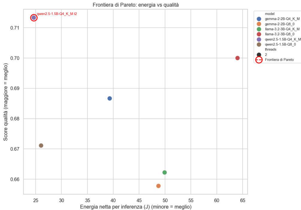
Figura 4.10: Frontiera di Pareto nel piano energia–qualità (Campagna A, i sei modelli a 2 thread; cerchiare in rosso le configurazioni non dominate).
