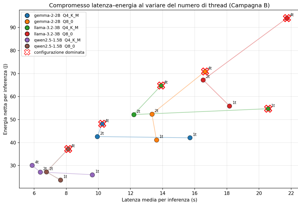
Figura 4.12: Compromesso latenza-energia al variare del numero di thread (Campagna B): per ogni modello è tracciata la traiettoria a 1, 2 e 4 thread e sono marcate in rosso le configurazioni dominate. I 4 thread risultano dominati in cinque modelli su sei.
