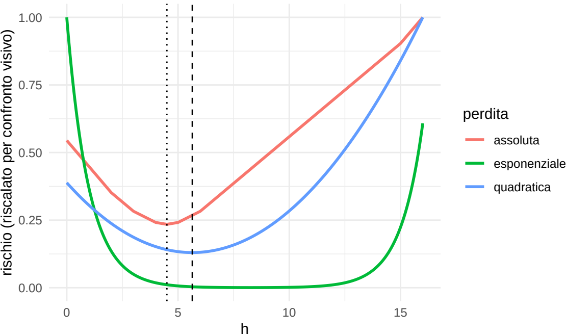
Rischio empirico al variare di h , per tre funzioni di perdita
