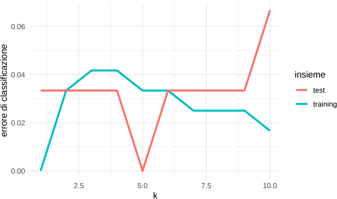
Errore KNN al variare di k, dataset Iris
