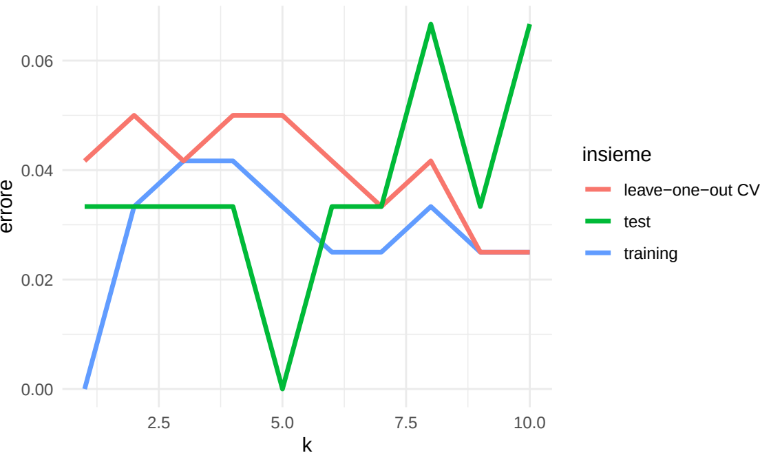
Errore KNN al variare di k : training, LOO-CV e test, dataset Iris
