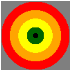
Bias: Basso – Varianza: Alta
