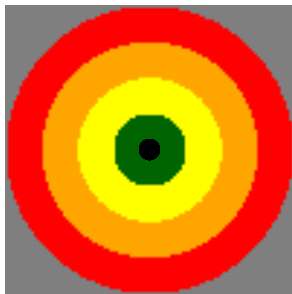
Bias: Basso – Varianza: Bassa
