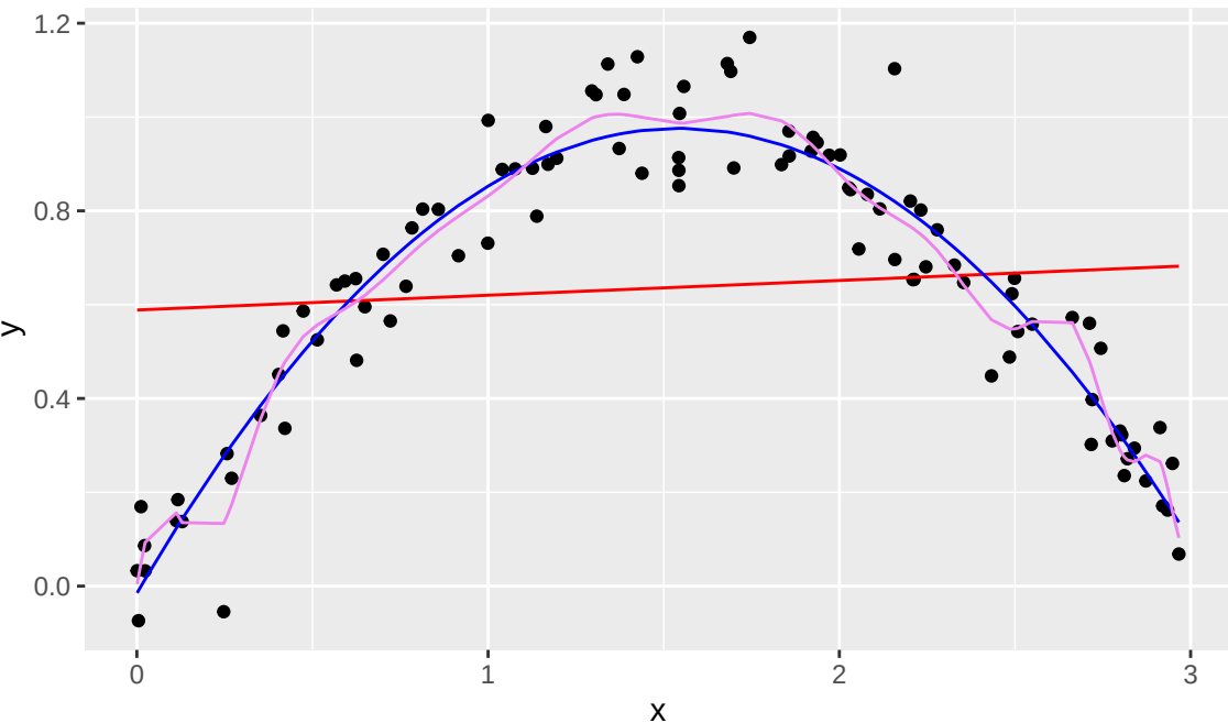
Regressione polinomiale di gradi 1 (rosso), 2 (blu), 30 (viola)
