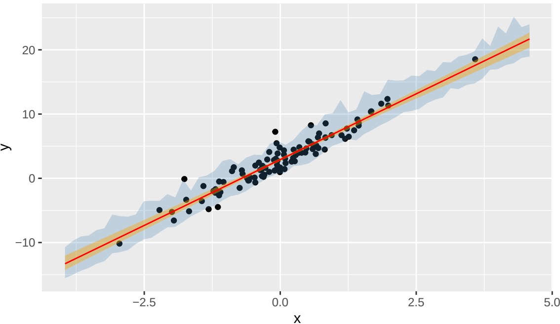
Bande di confidenza (arancione) e di previsione (blu) bootstrap
