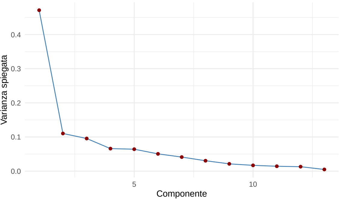
Scree plot – componenti principali di Boston
