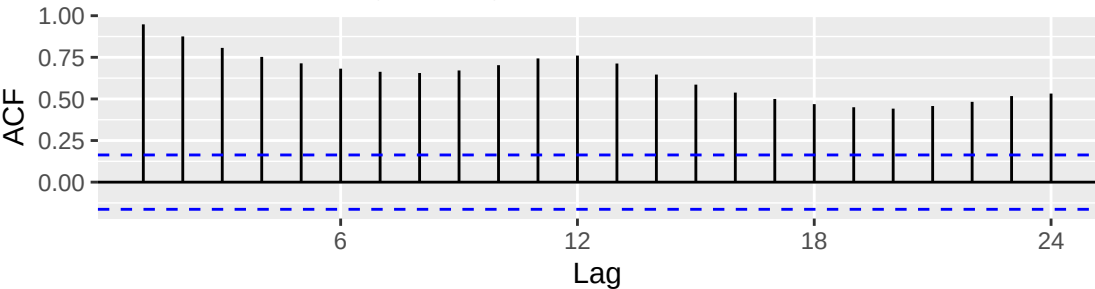
ACF di AirPassengers originale
