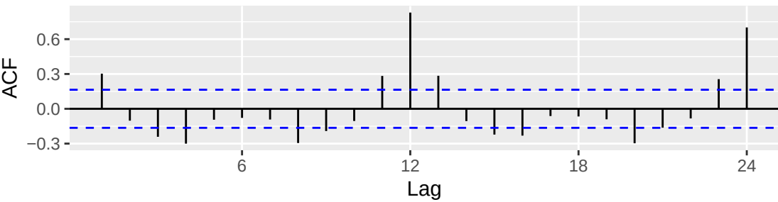
ACF di AirPassengers differenziata
