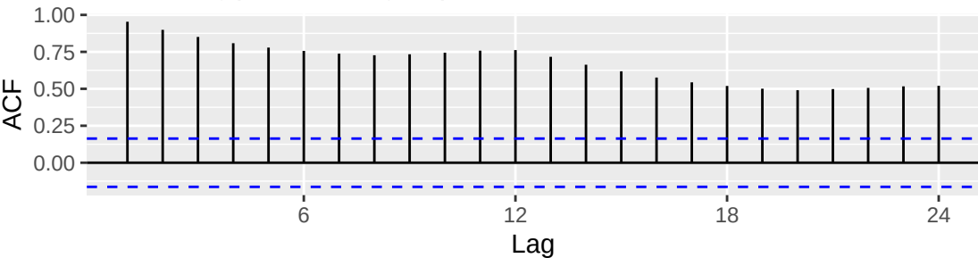
ACF di \log(\text{AirPassengers})
