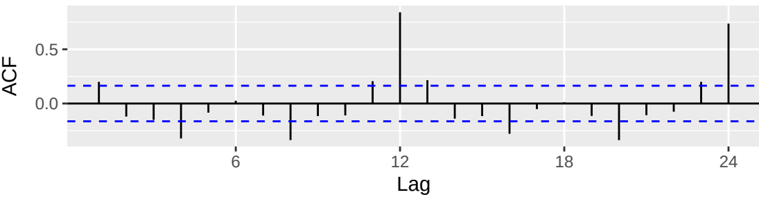
ACF della differenza del logaritmo
