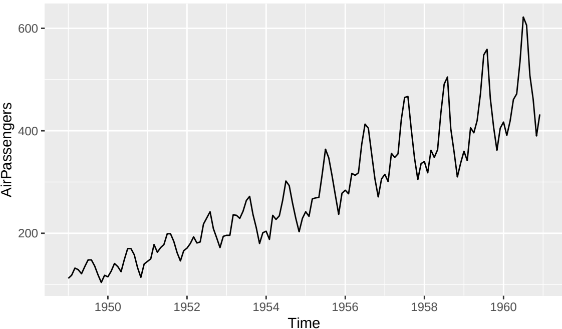
Serie AirPassengers
