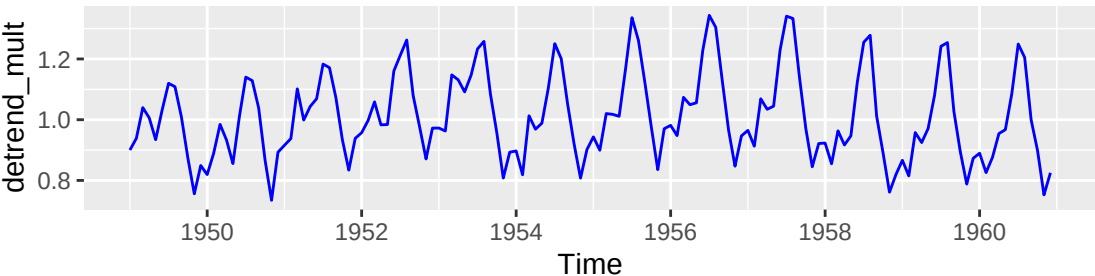
Serie detrendizzata (moltiplicativa)
