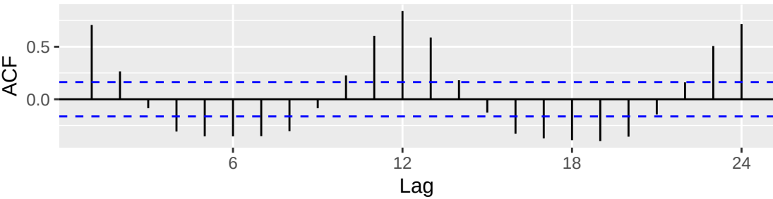
ACF della serie detrendizzata (esponenziale)
