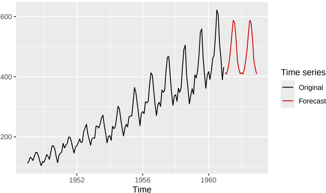
Previsione KNN per AirPassengers (lag 1:12, k=3)
