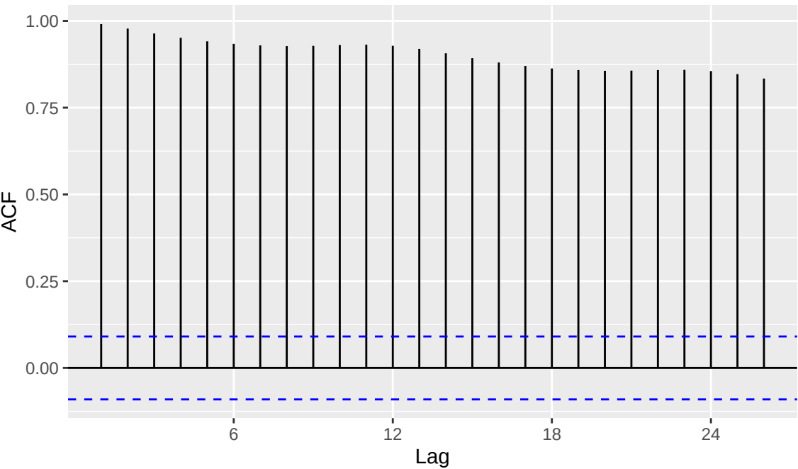
Series: co2
