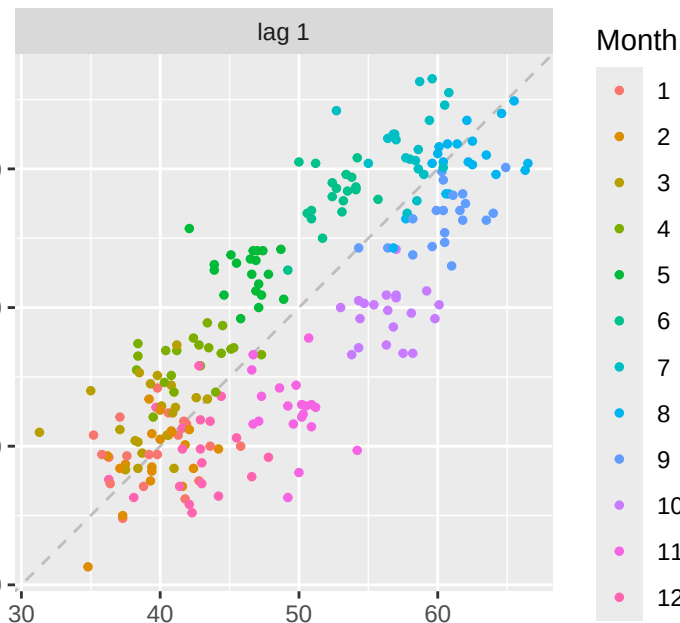
Lag plot di nottem, k = 1
