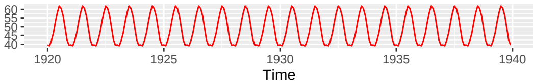
Componente stagionale stimata
