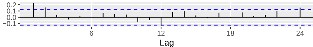
ACF dei residui
