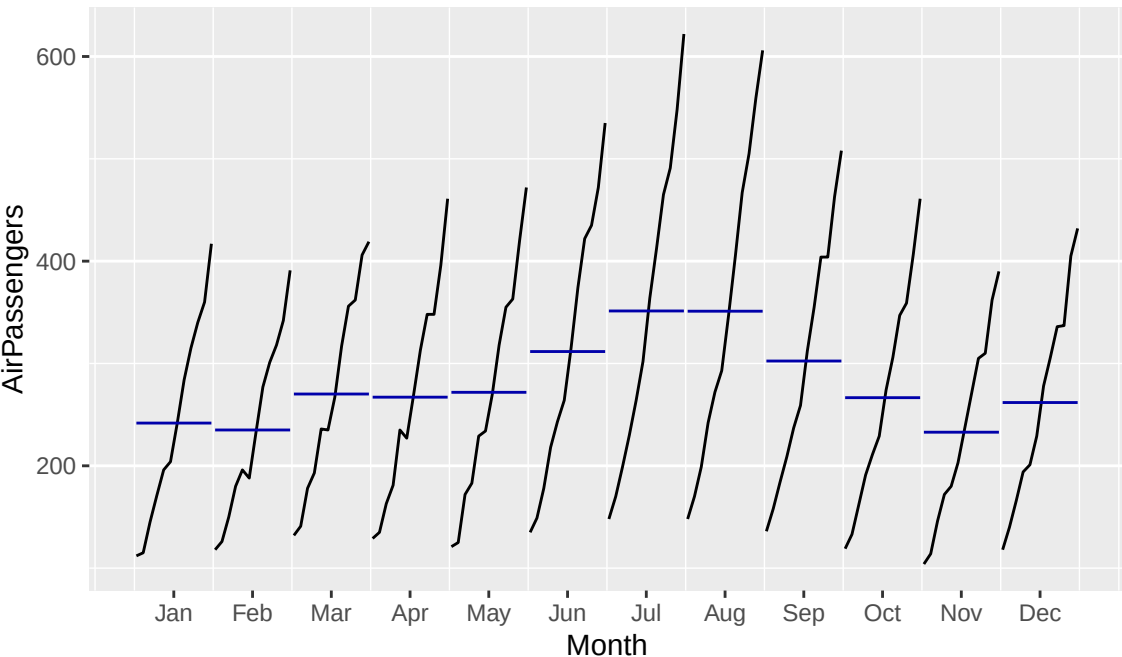
AirPassengers: grafico stagionale di sottoserie
