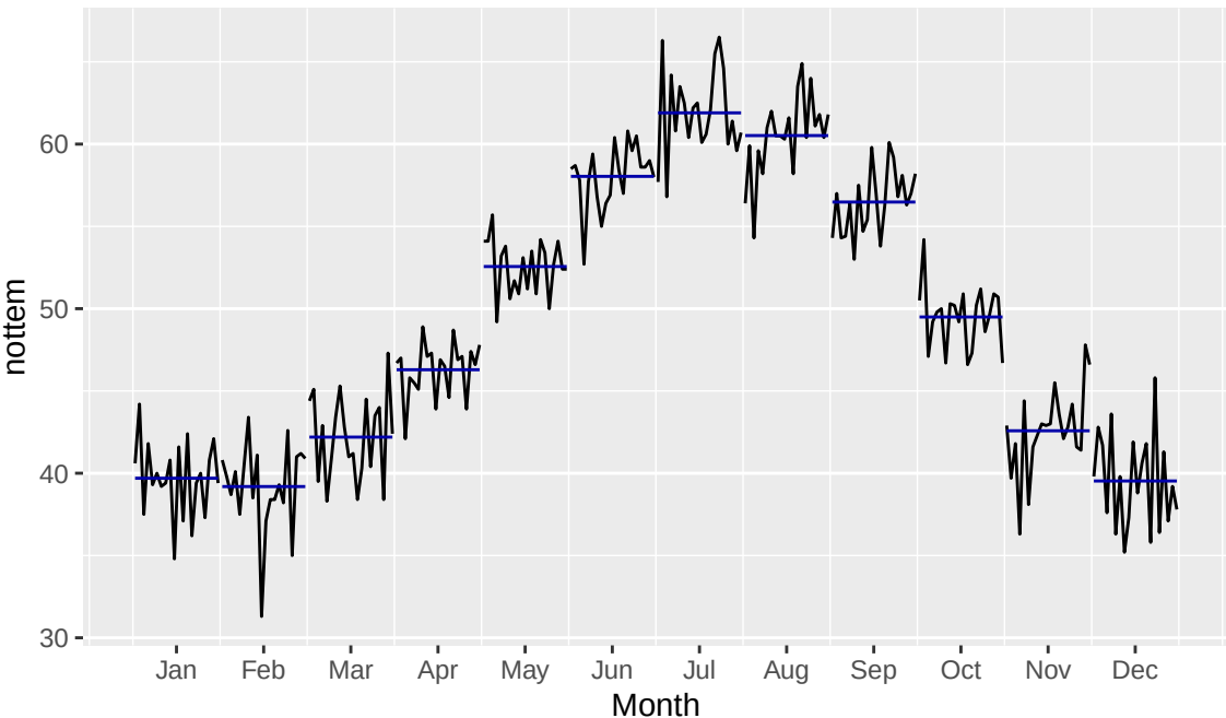
nottem: grafico stagionale di sottoserie
