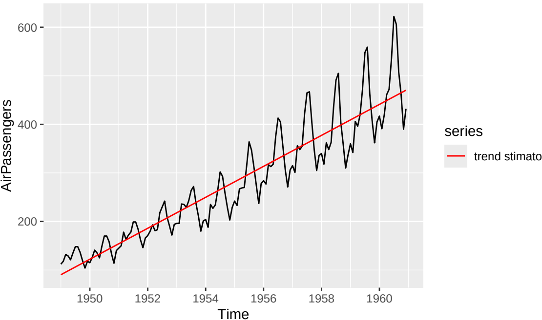
AirPassengers e trend stimato (lineare)
