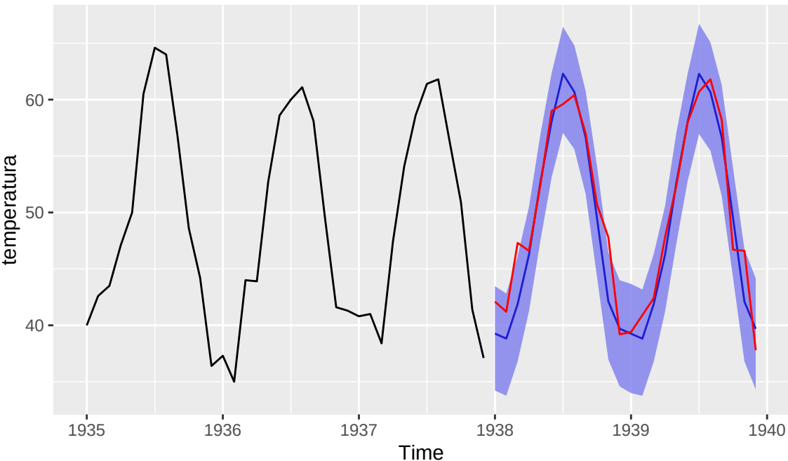
Intervalli di previsione bootstrap al 95%, ETS(A,A,A), nottem
