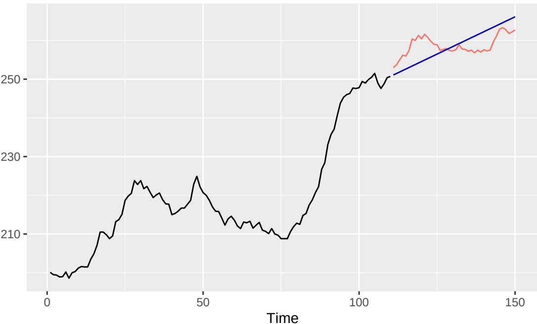
Modello di Holt, serie BJsales
