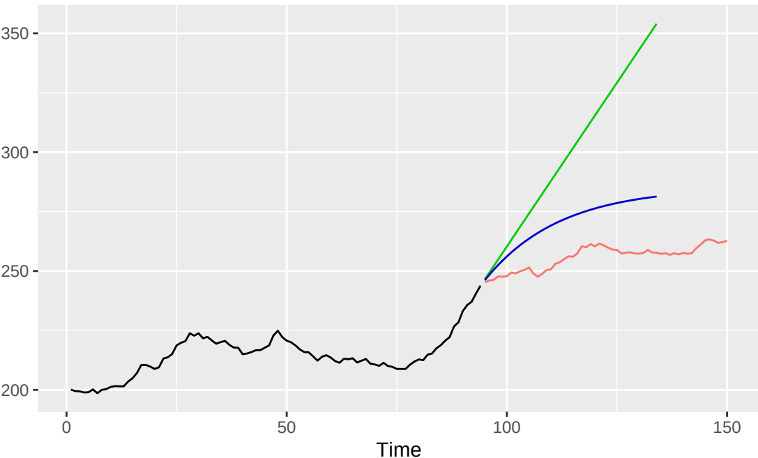
Holt senza damping (verde) vs con damping (blu), BJsales
