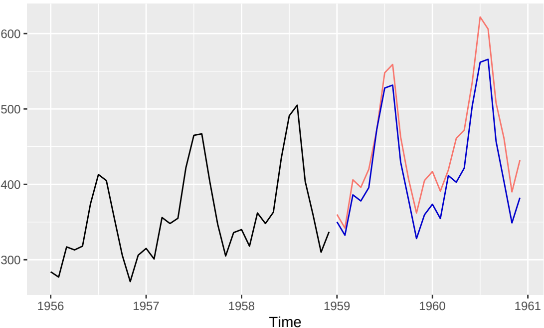
Holt-Winters con stagionalità moltiplicativa, serie AirPassengers
