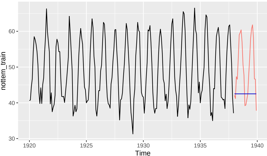
SES con alpha = 0.5, serie nottem
