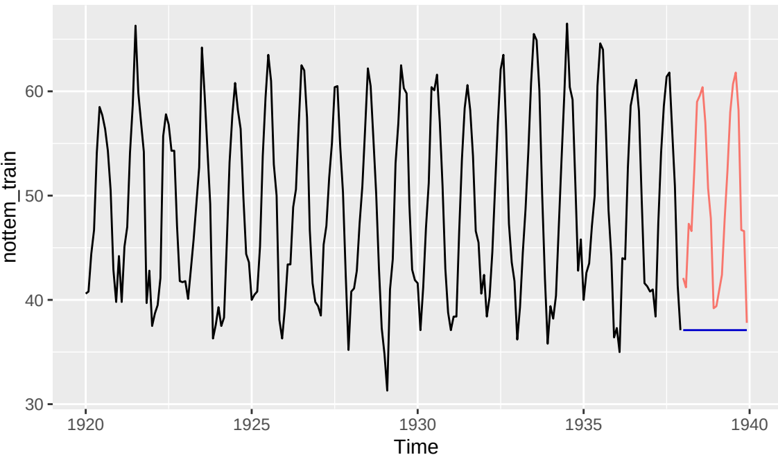
SES con \alpha = 1 (equivalente al naive), serie nottem
