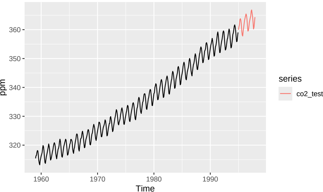
Concentrazione di CO2 atmosferica, serie co2 (training)
