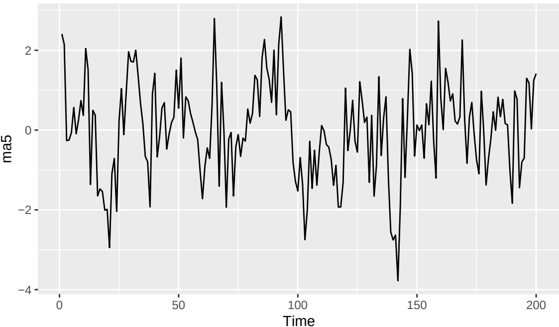
MA(5) simulato
