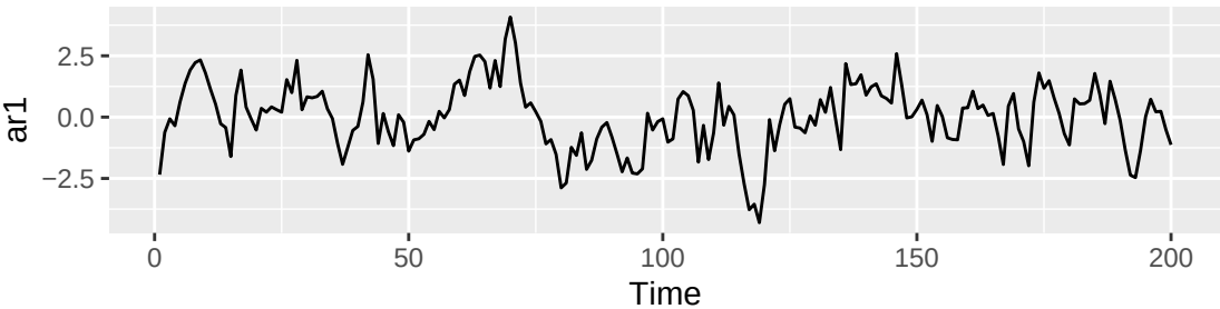
AR(1)
