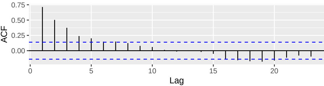
ACF
