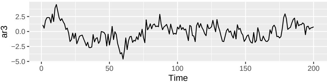
AR(3)
