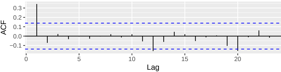
ACF
