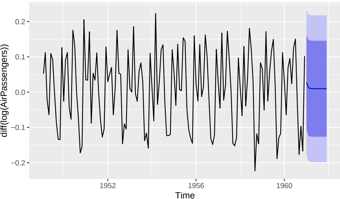
Previsione AR(1), intervalli parametrici
