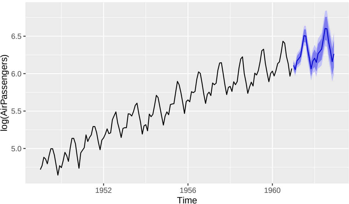
Previsione con auto.arima() su log(AirPassengers)
