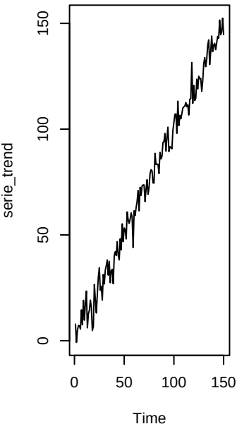
Trend + rumore
