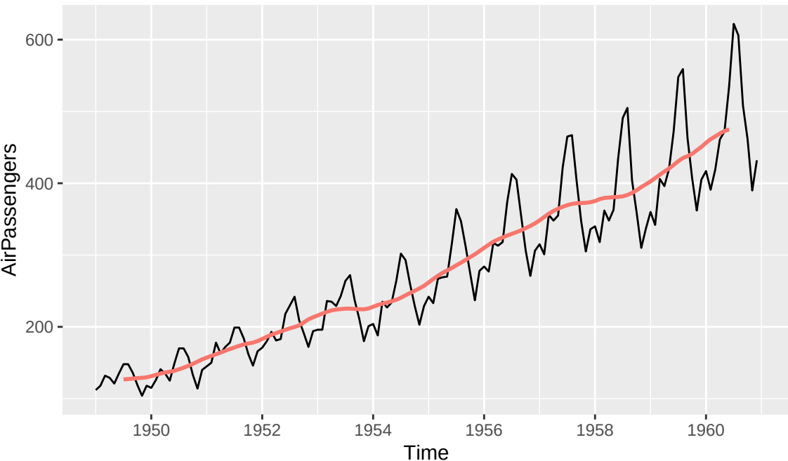
AirPassengers e trend stimato con media mobile
