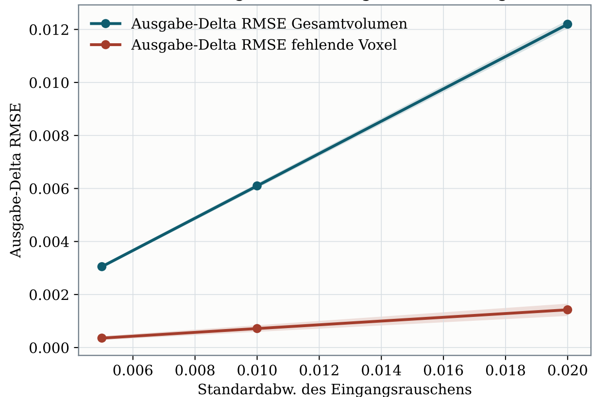
Änderung der Vorhersage unter Störung
