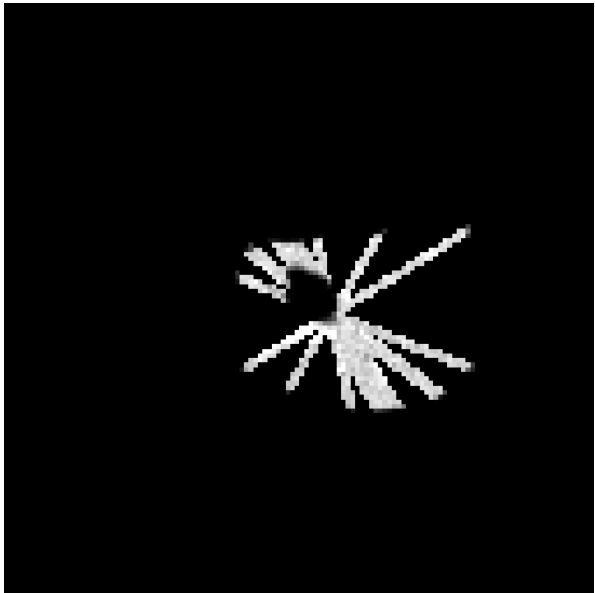
Sparse Volume
