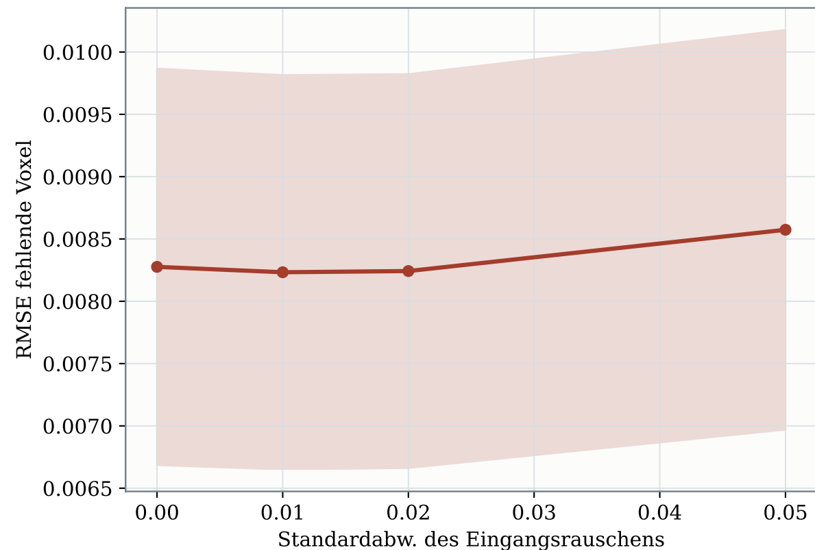
Eingabesensitivität
