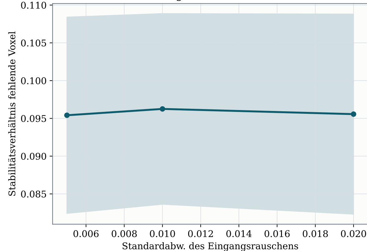
Eingabesensitivität
