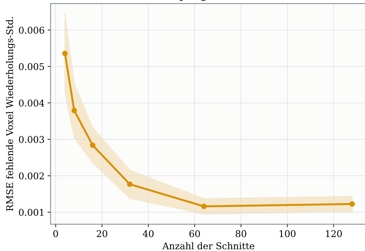
Sampling-Stabilität
