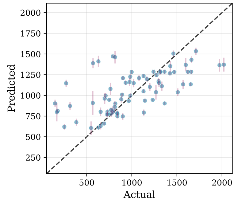
SBЭТ, м2/г R^2=0.378 , RMSE=329.47
