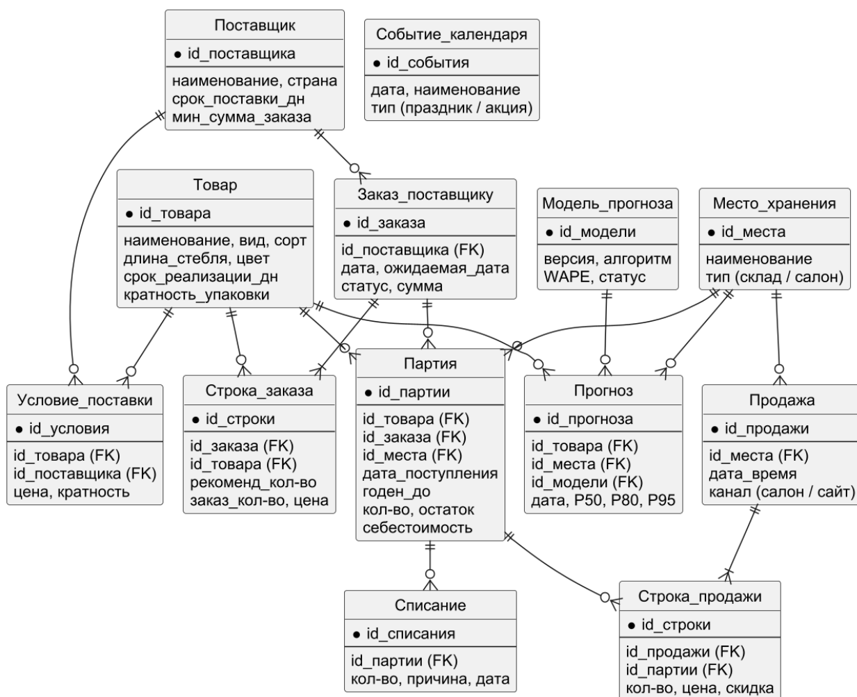
Рисунок 4.3 – Информационная модель системы (диаграмма «сущность–связь»)
