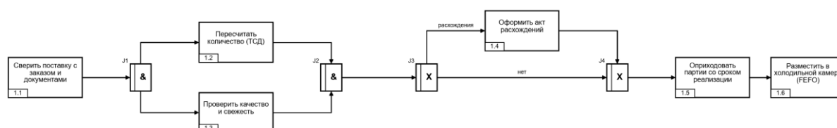
Рисунок 5.4 – Диаграмма IDEF3 декомпозиции блока А1
