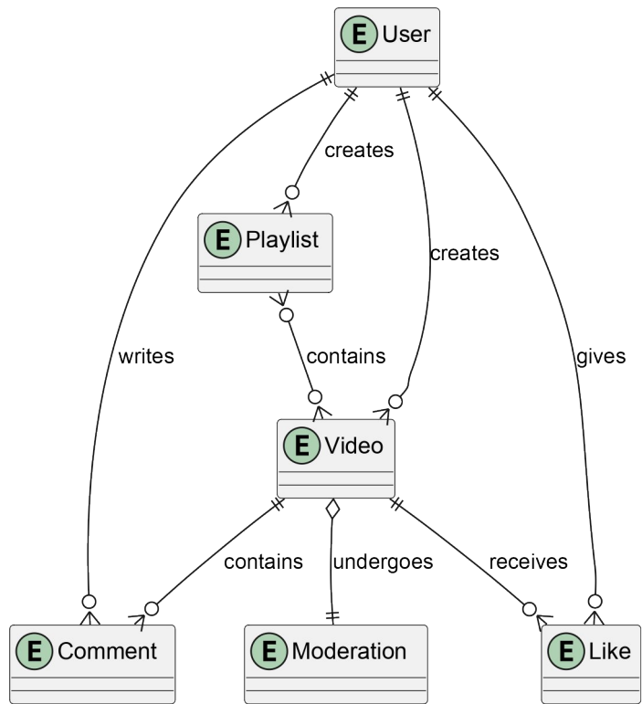
Рисунок 1 – Диаграмма ассоциаций между сущностями видеохостинга
