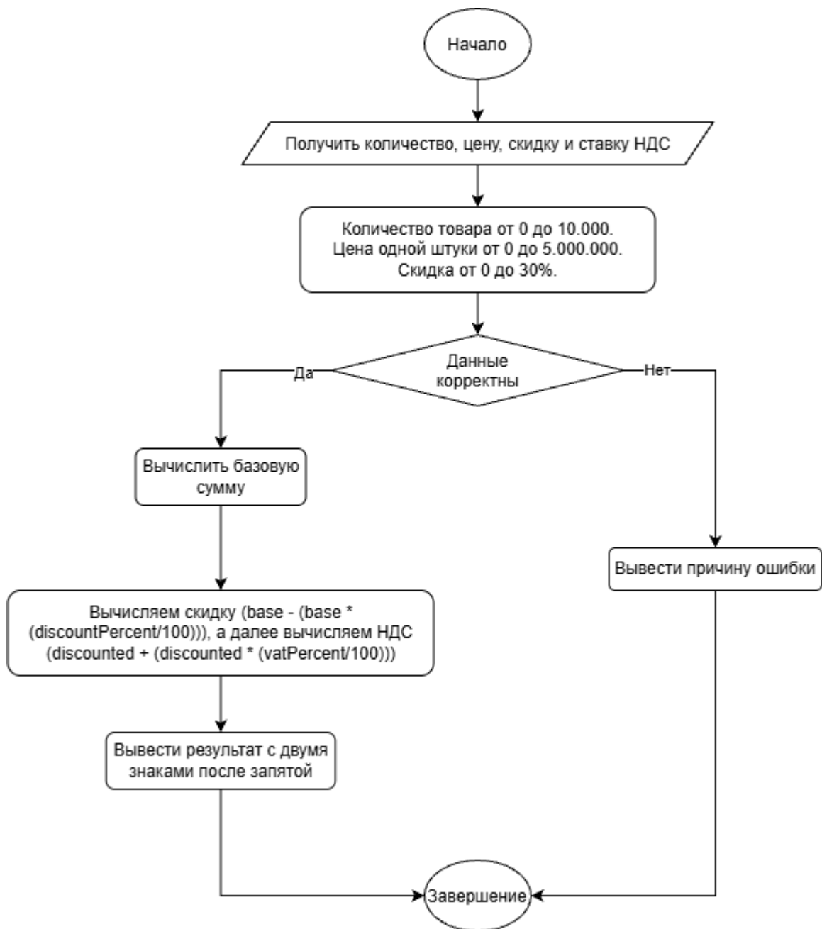
Рисунок 1 — Activity-диаграмма для практической работы 1
