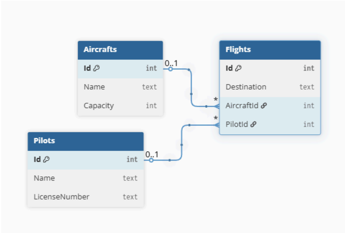
ERD-діаграма БД:
