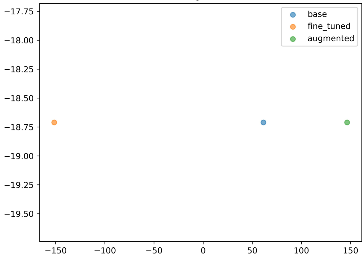
Digit 2
