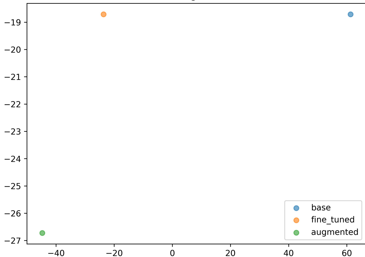
Digit 3
