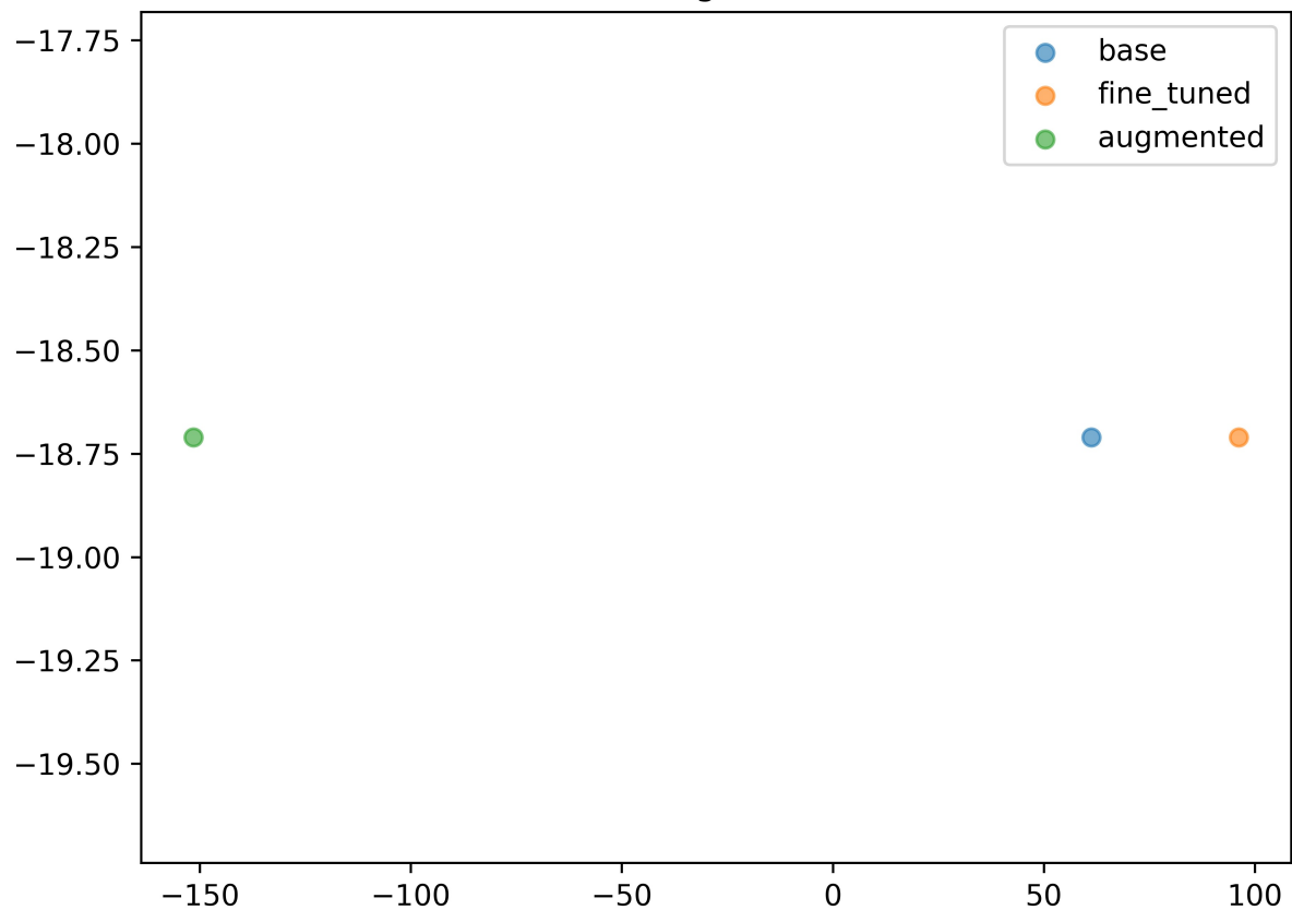
Digit 4
