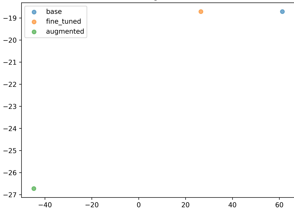
Digit 9
