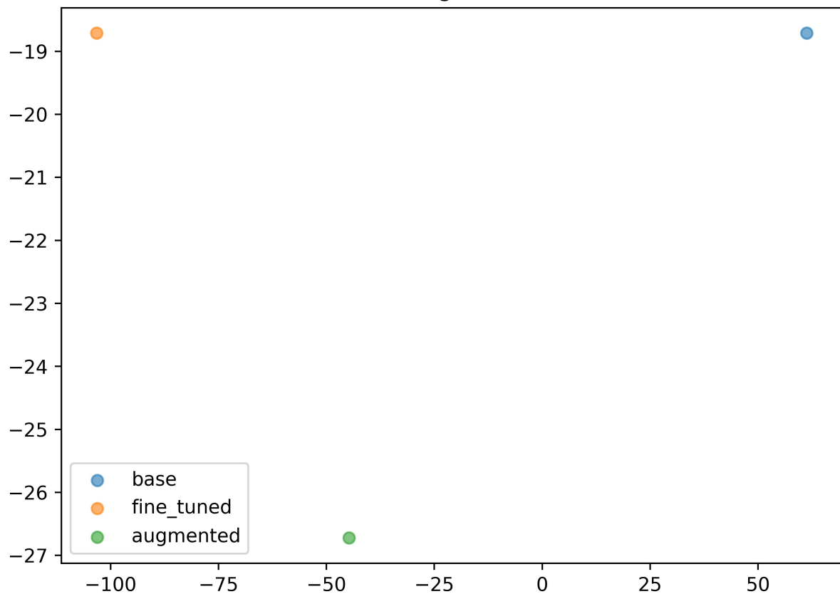
Digit 7
