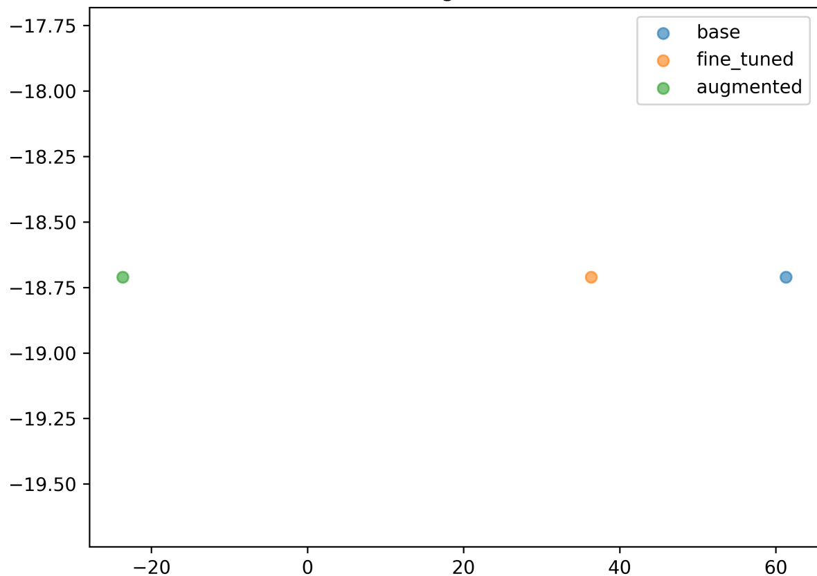
Digit 6
