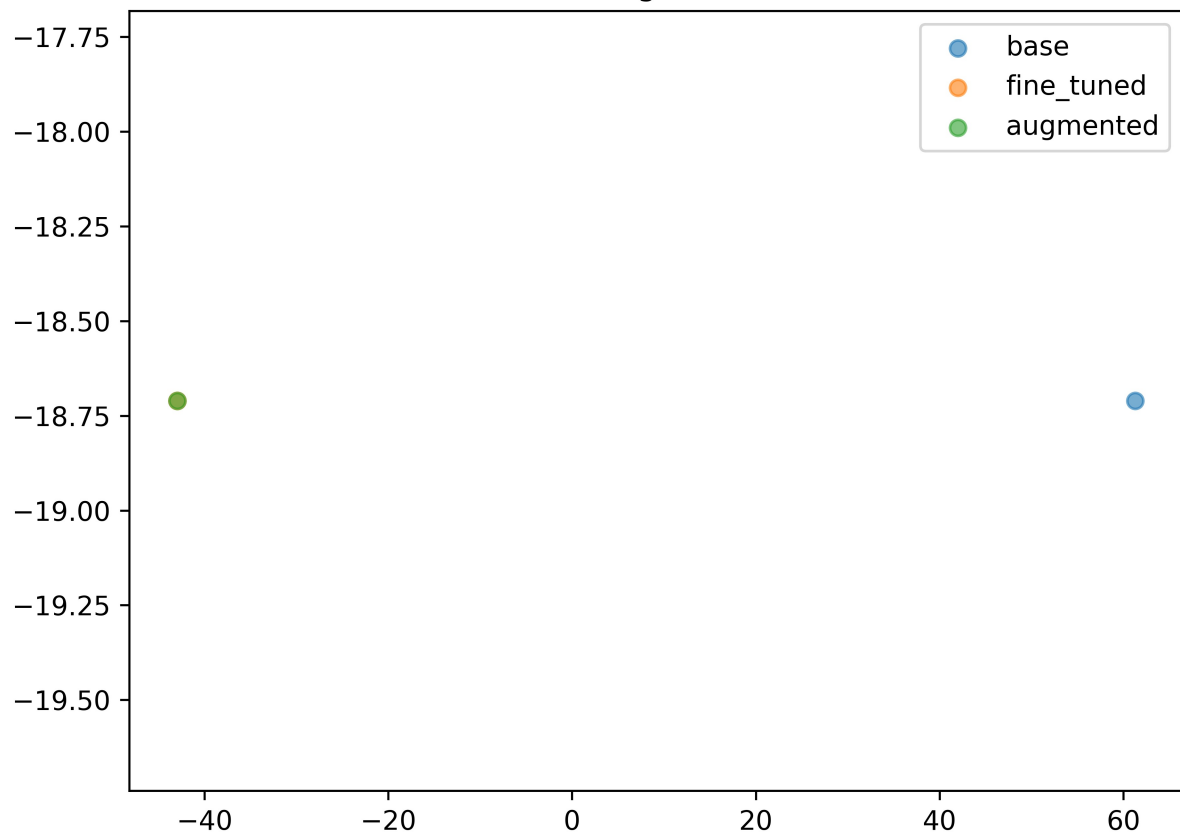
Digit 0
