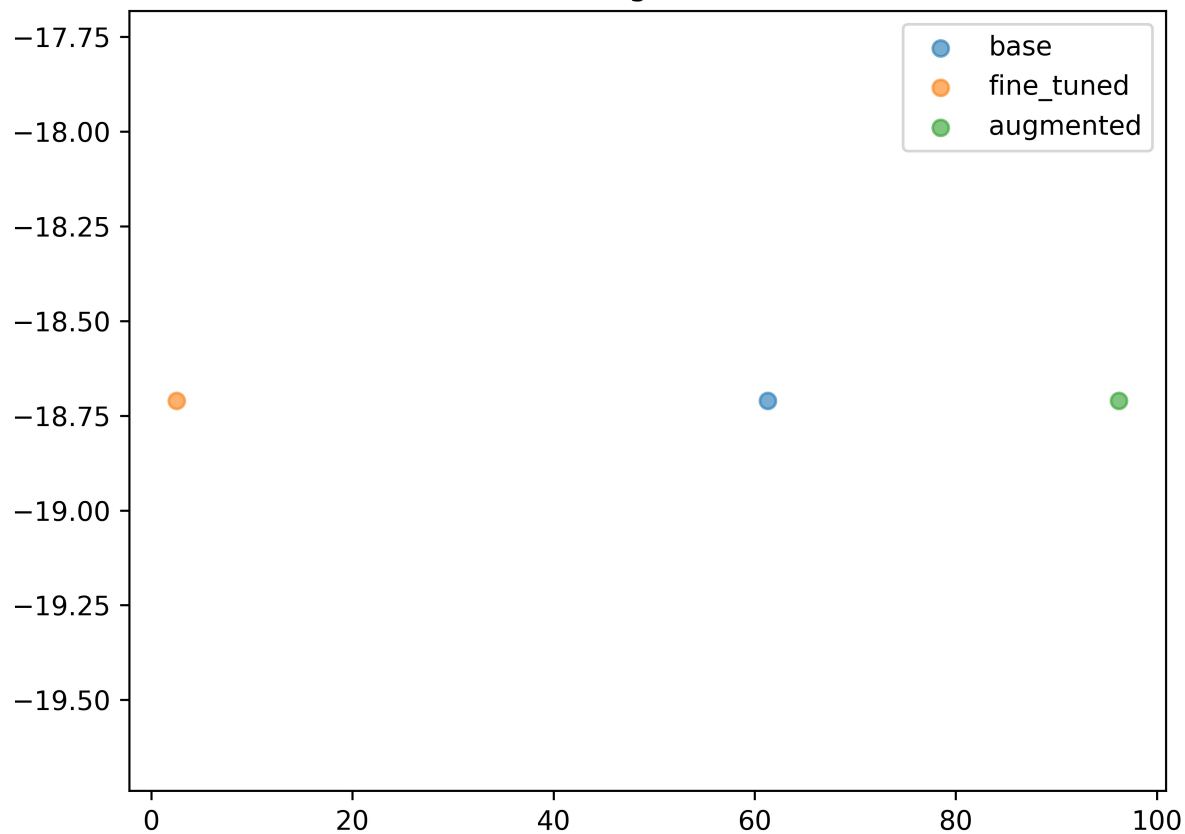
Digit 8
