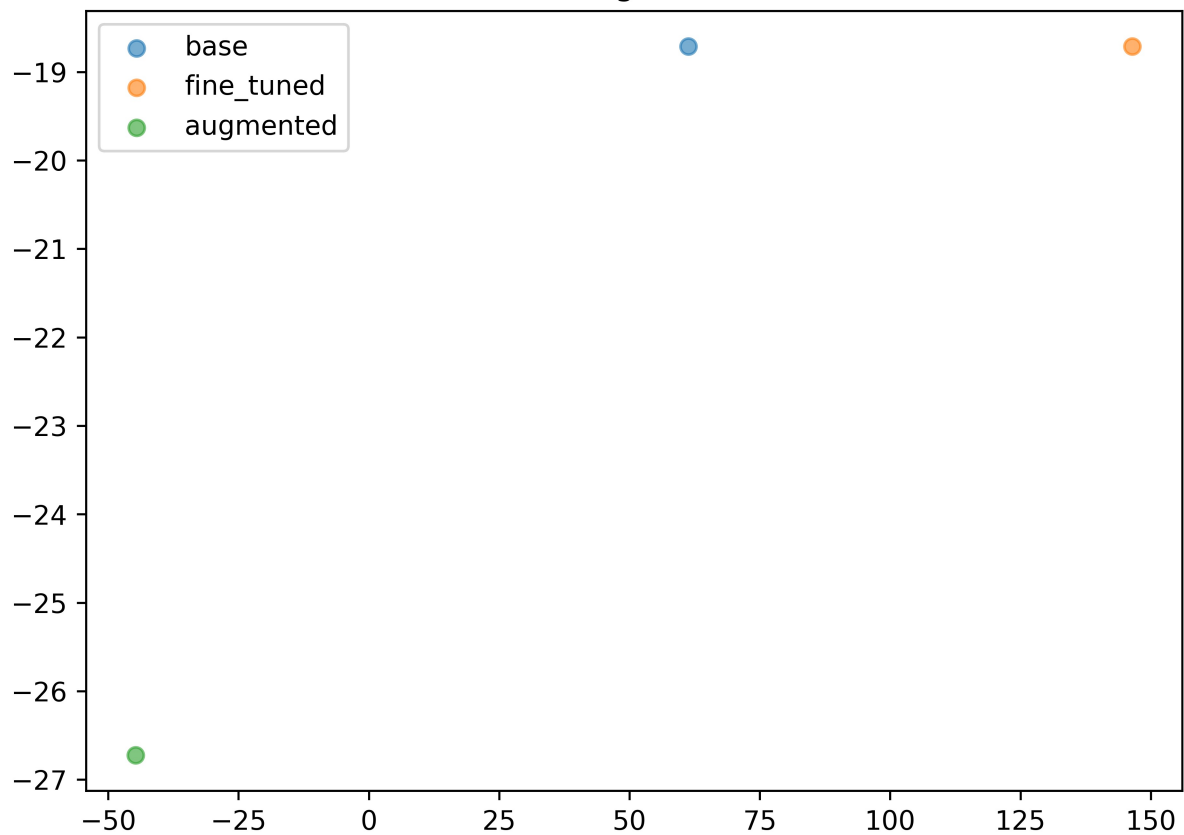
Digit 1
