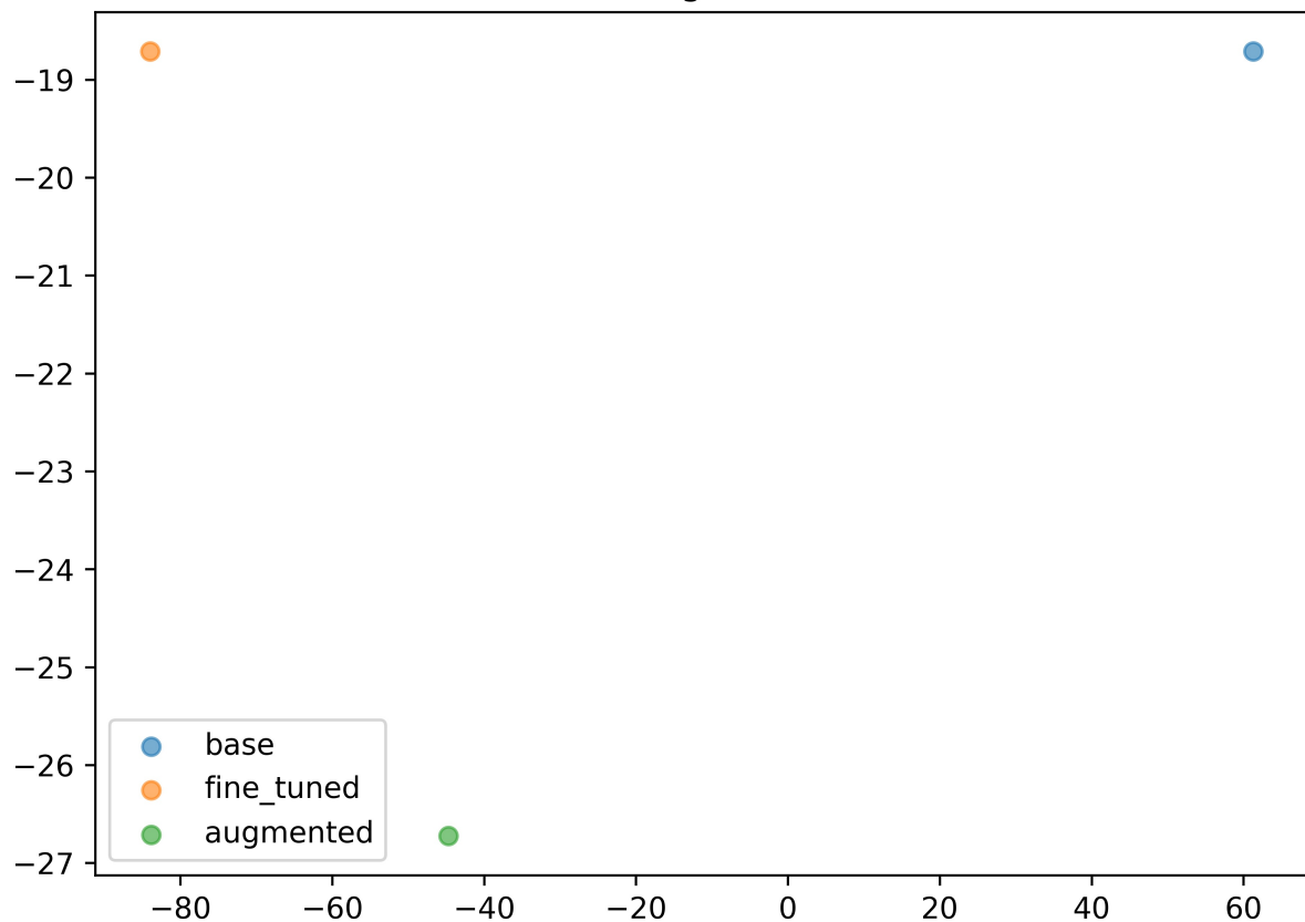
Digit 5
