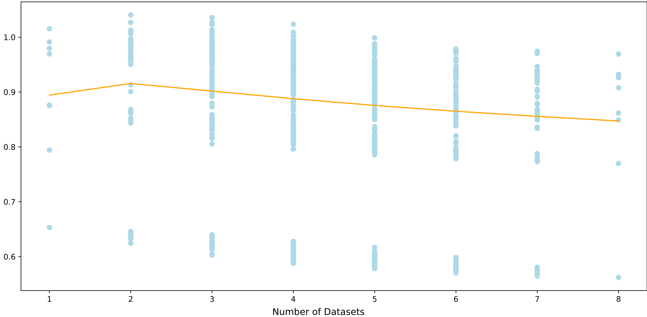
Layer 11
