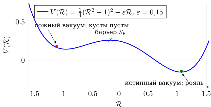
Рис. 1: Потенциал рояльного поля. Точки минимумов и максимума получены решением V'(R) = R^3 - R - \varepsilon = 0 при \varepsilon = 0,15 : R = -1,0742 ; -0,1483 ; 1,0742 . Разность глубин 2\varepsilon R_0 = 0,322 соответствует выигрышу в числе доступных сюжетов.
