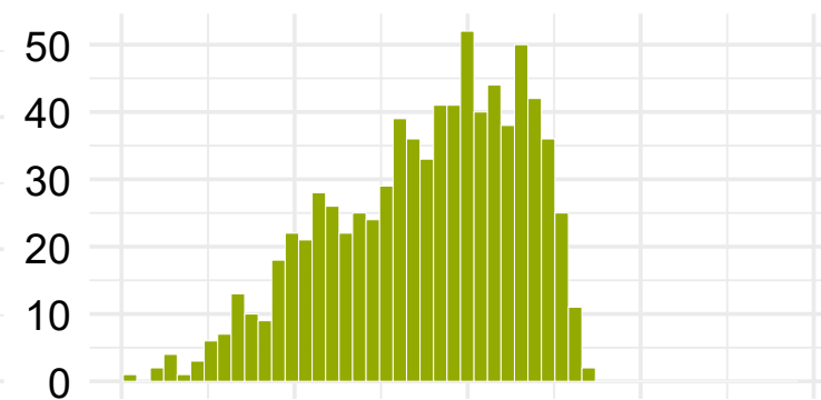
Top 100
