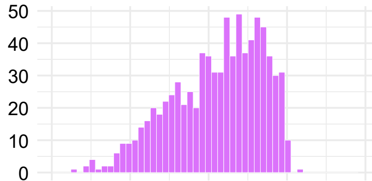
Top 50
