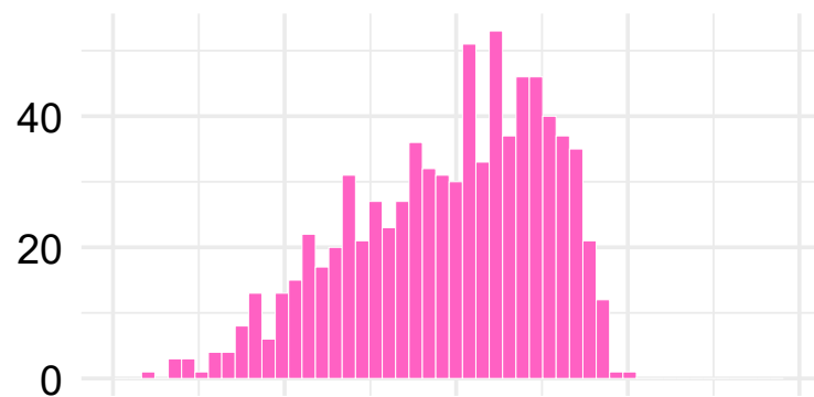
Top 70
