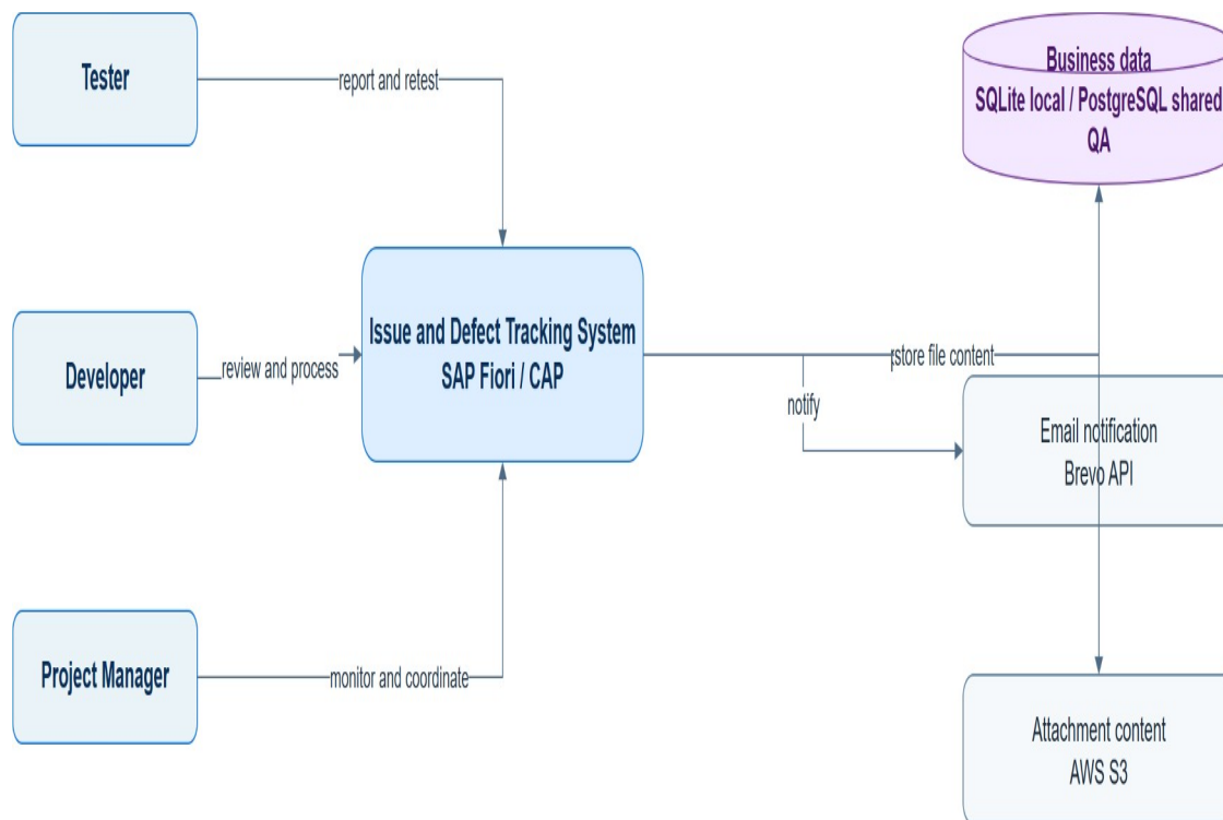
Figure 01. System Context. IDTS Diagram Pack; bản có thể chỉnh sửa được quản lý dưới dạng file draw.io cùng artifact của dự án.
