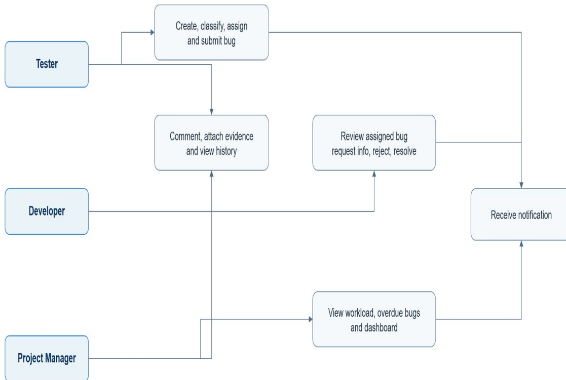
Figure 03. Use Case Diagram. IDTS Diagram Pack; bản có thể chỉnh sửa được quản lý dưới dạng file draw.io cùng artifact của dự án.
